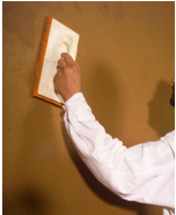
Abbildung 6.1.8: Oberflächenbearbeitung von Lehm-Oberputz fein durch Reiben mit dem Schwamm Brett
