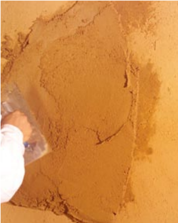
Abbildung 6.1.5: Auftrag von Lehm-Oberputz grob mit dem Edelstahlglätter, Auftragsstärke ca. 1 cm
